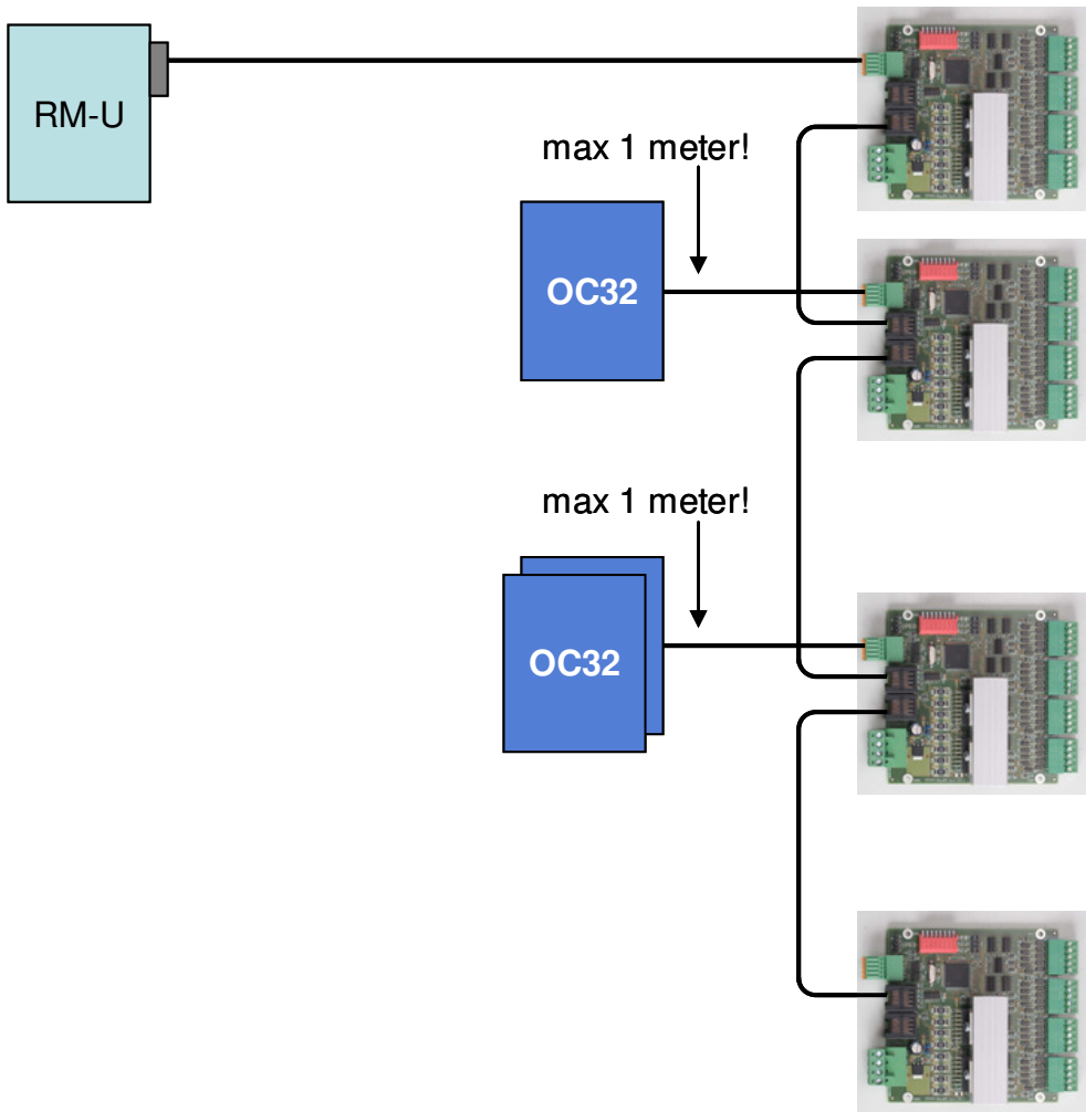
Fig 14: Netwerkbewrading tussen Dinamo modules, voorbeeld methode 2
