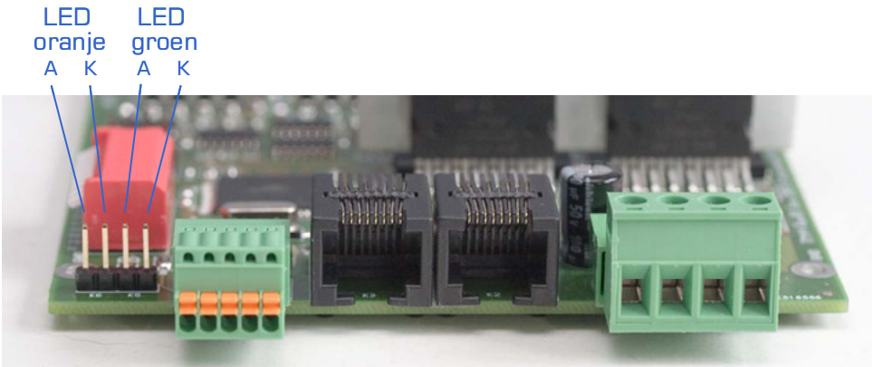
Fig 17: Externe aansluiting LEDs
