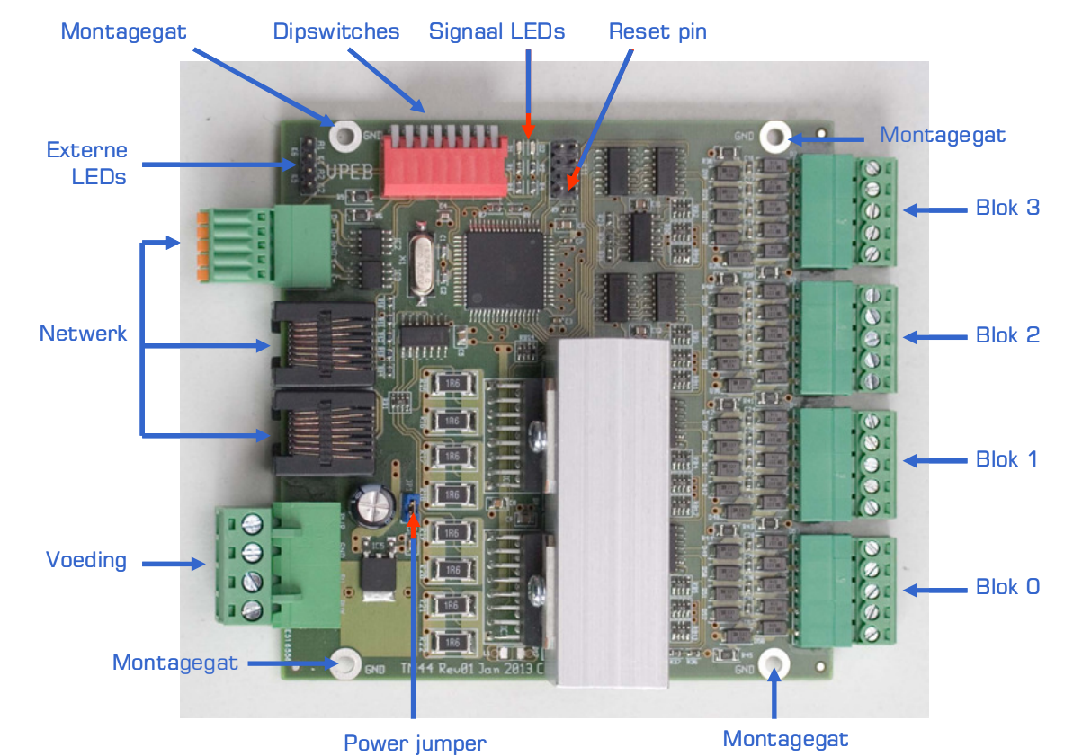
Fig 2: Opbouw en functies TM44
