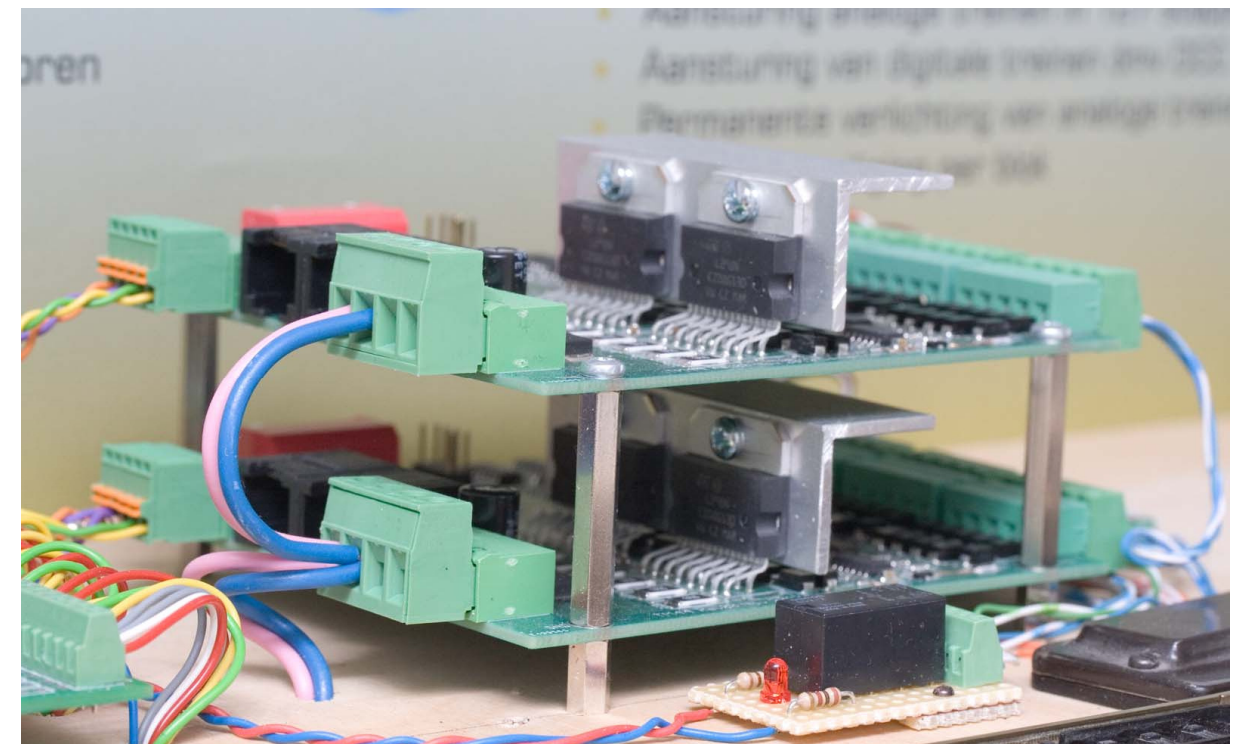
Fig 3: Montage meerdere TM44's
