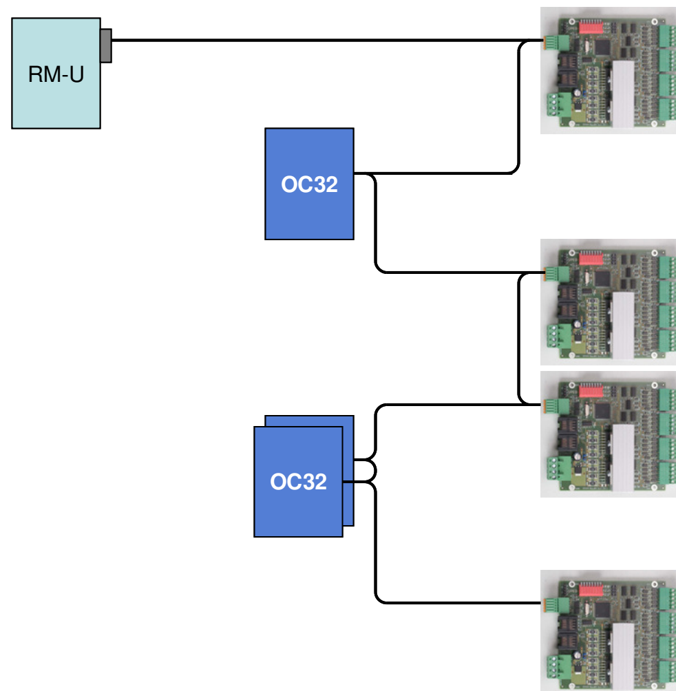
Fig 13: Netwerkbedrading tussen Dinamo modules, voorbeeld methode 1
